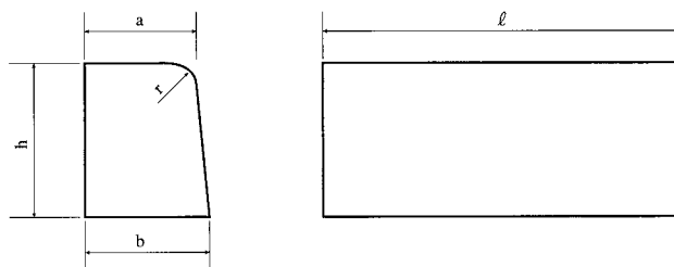
片面歩車道境界ブロック
