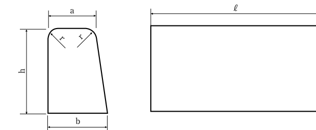
駒止めブロック
