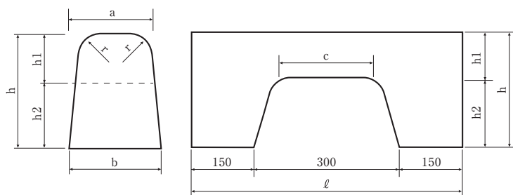
両面歩車道境界ブロック
