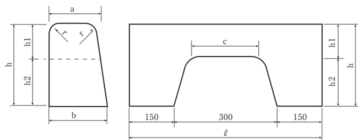
駒止めブロック
