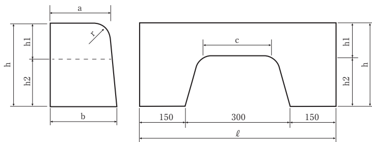
片面歩車道境界ブロック
